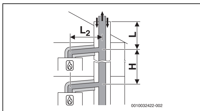
Rys. 28 Wykorzystanie wielokrotnie wg C_{(14)3x} ze wspólnym sztywnym odprowadzeniem spalin i koncentryczną instalacją powietrzno-spalinową w pomieszczeniu zainstalowania
