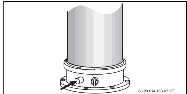
Rys. 46 Króciec pomiarowy spalin
