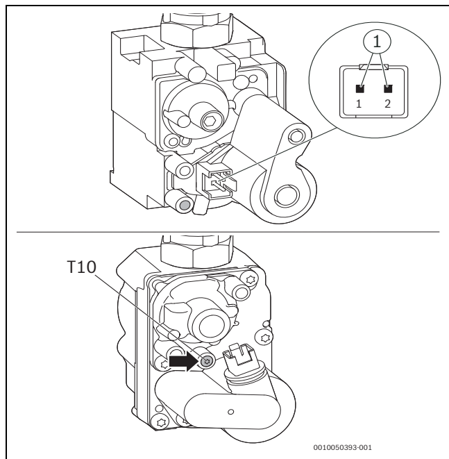
Rys. 50 Punkty pomiarowe na armaturze gazowej
