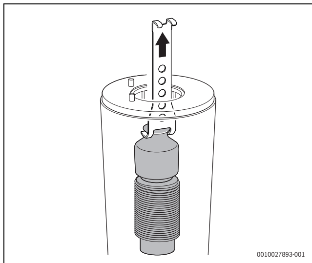
Rys. 58 Wyjmowanie górnego elementu waporowego
