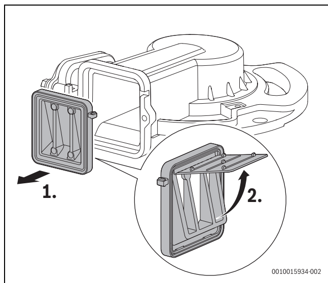
Rys. 56 Zabezpieczenie przed przepływem zwrotnym w urządzeniu mieszającym
