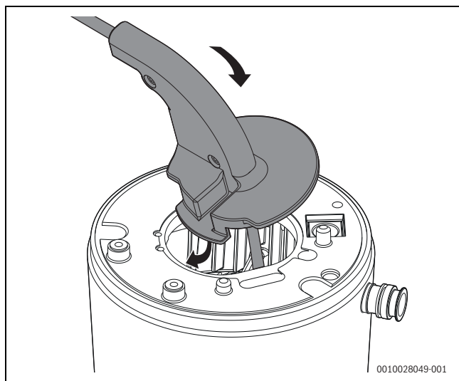
Rys. 60 Umieszczanie szczotki w bloku ciepłym
