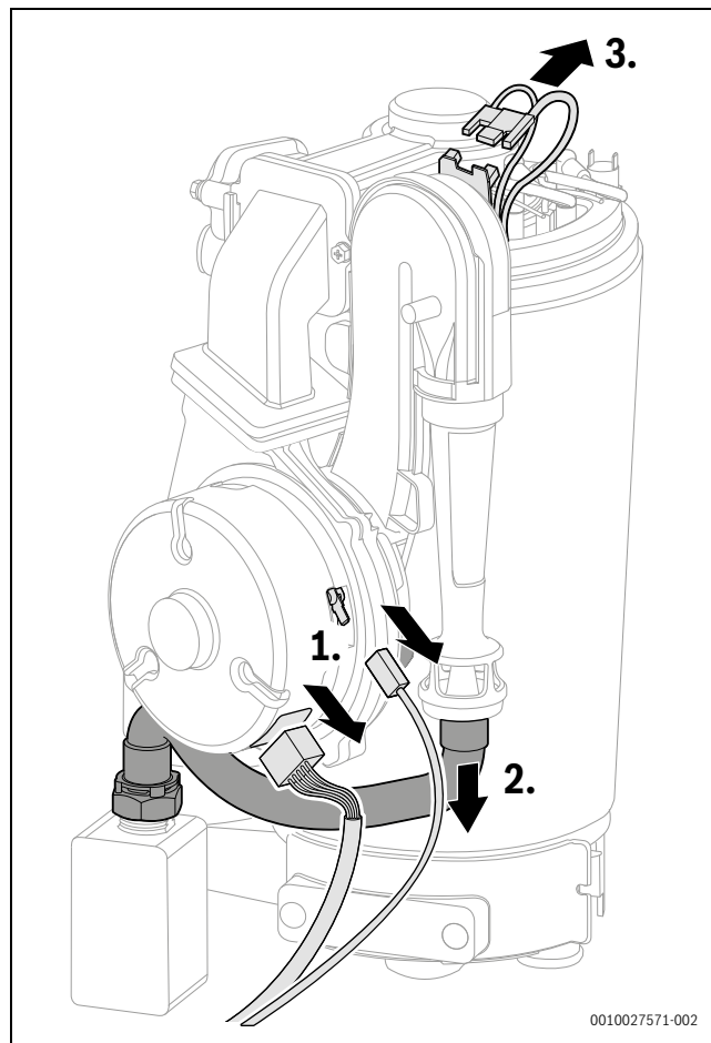
Rys. 51 Odłączanie wtyczki i węża gazu
