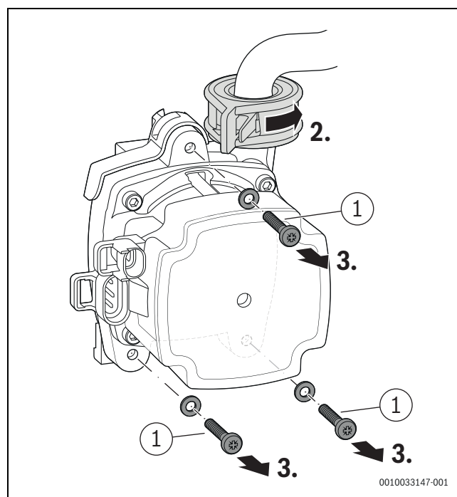
Rys. 69 Odblokowanie pompy c.o. i usuwanie śrub
