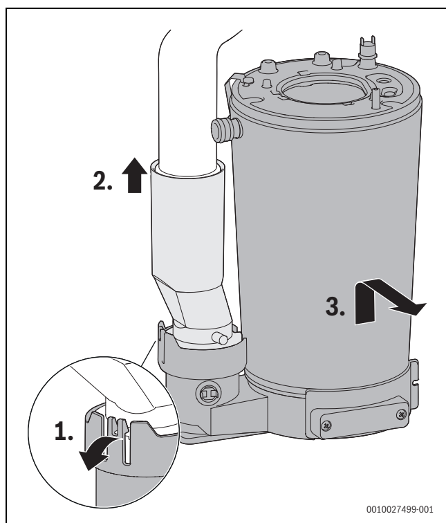
Rys. 67 Demontaż bloku cieplnego
