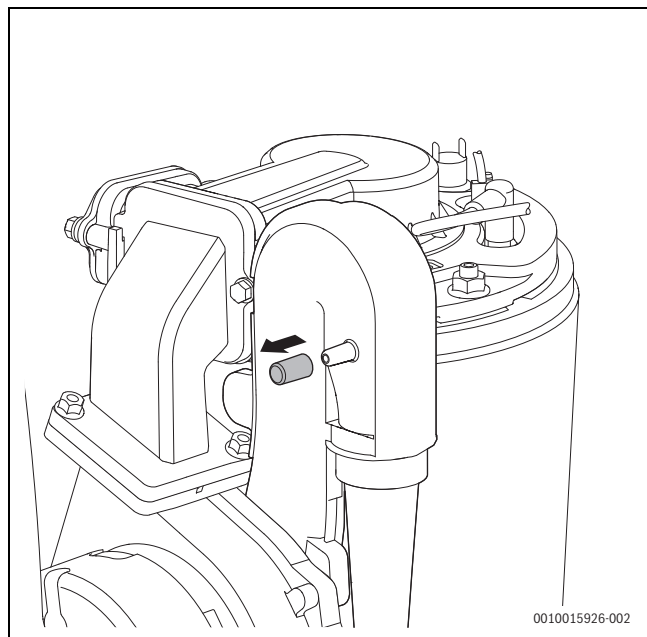
Rys. 49 Króciec pomiarowy na zespole mieszającym
