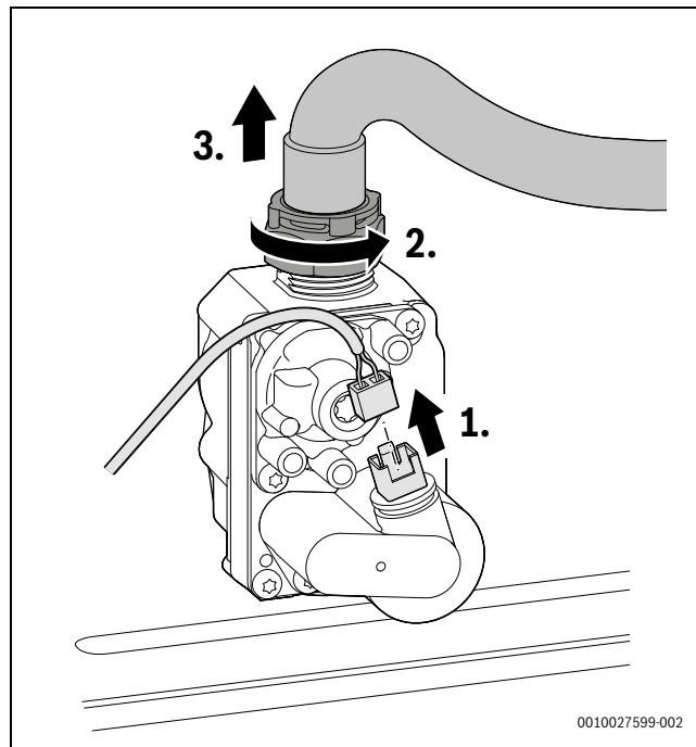
Rys. 72 Odłączanie wtyczki od armatury gazowej i usuwanie nakrętki z węzłem gazowym
