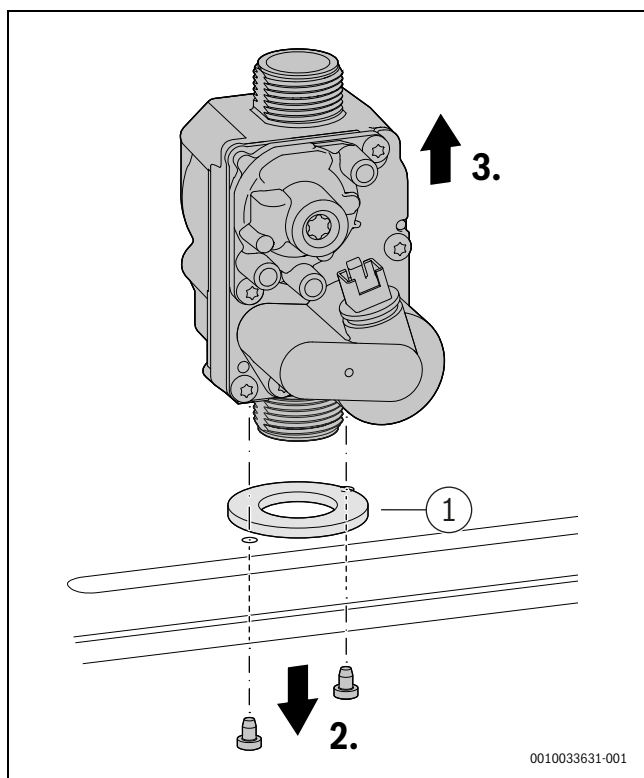
Rys. 75 Demontaż armatury gazowej
