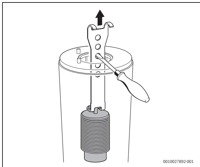
Rys. 59 Wyjmowanie dolnego elementu wyporowego
