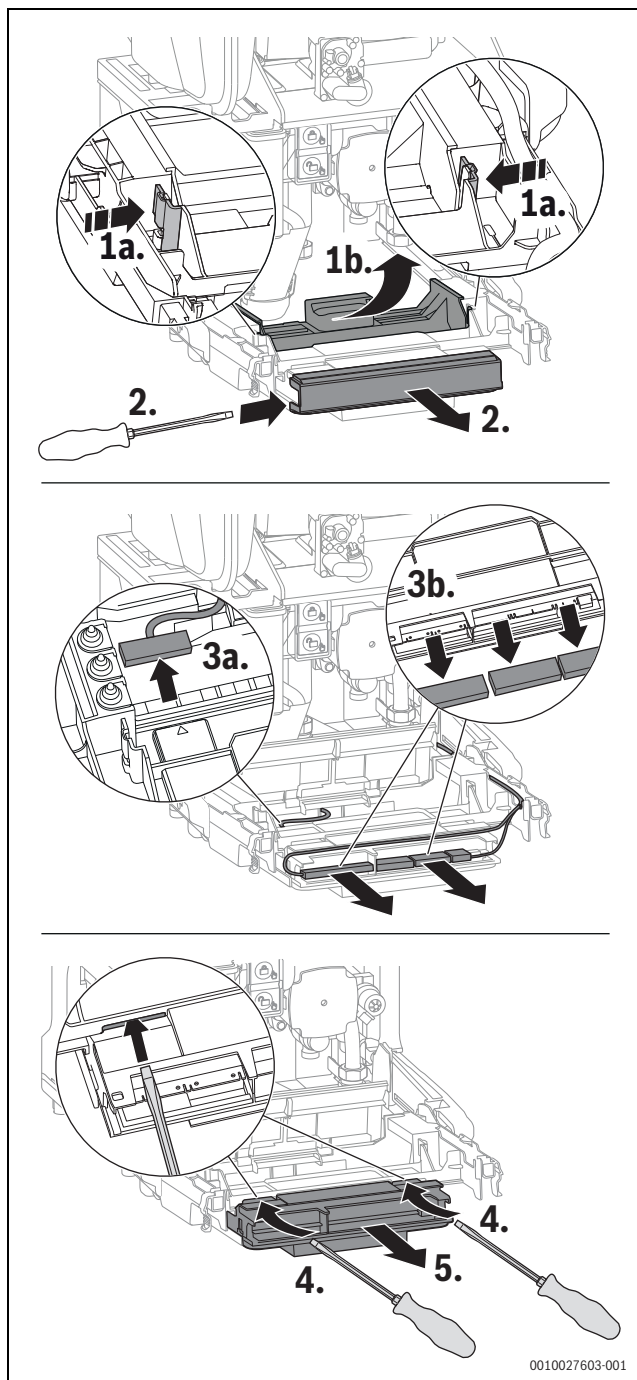
Rys. 80 Wyjmowanie sterownika
