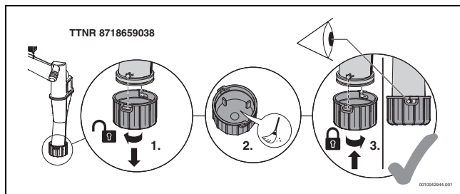
Rys. 82 Czyszczenie osadnika zanieczyszczeń
