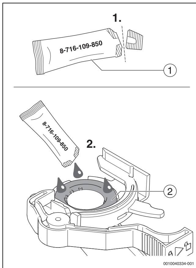
Rys. 84 Smarowanie uszczelki
