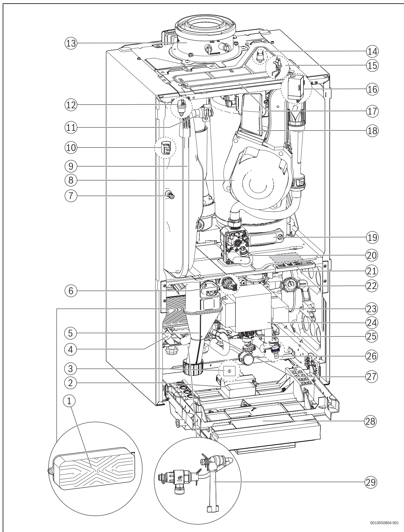
Rys. 6 Przegląd produktu
