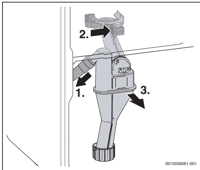
Rys. 81 Demontaż syfonu kondensatu
