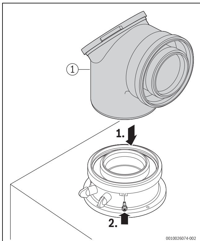
Rys. 38 Wkładanie osprzętu spalinowego i zabezpieczanie go śrubą
