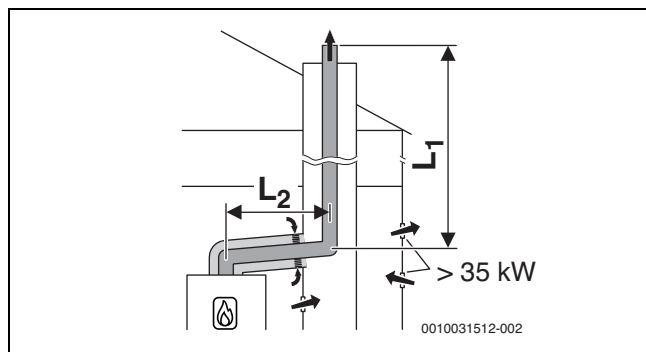
Rys. 24 Sztynne odprowadzenie spalin w szachcie wg B 33 z zależnym od powietrza w pomieszczeniu doprowadzeniem powietrza przez koncentryczną instalację powietrzno-spalinową w pomieszczeniu zainstalowania
