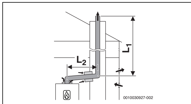
Rys. 22 Sztywne prowadzenie spalin w szachcie zgodnie z B 53p z dopływem powietrza zależnym od powietrza w pomieszczeniu przy urządzeniu i koncentrycznej złączce między pomieszczeniem instalacyjnym a szachtem
