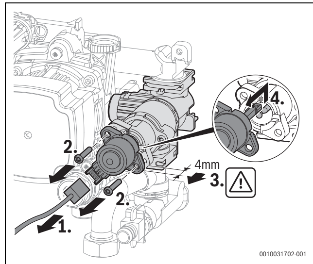
Rys. 88 Demontaż napędu zaworu 3-drogowego (wariant ze śrubami)
