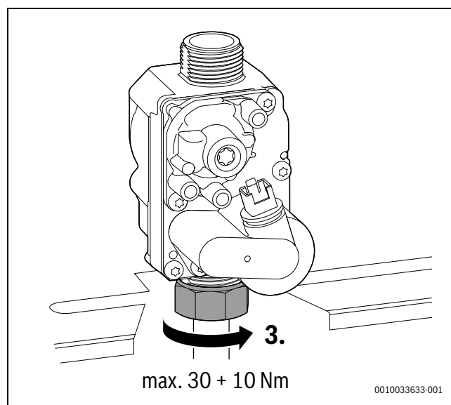
Rys. 77 Przestrzeganie momentu dokręcenia
