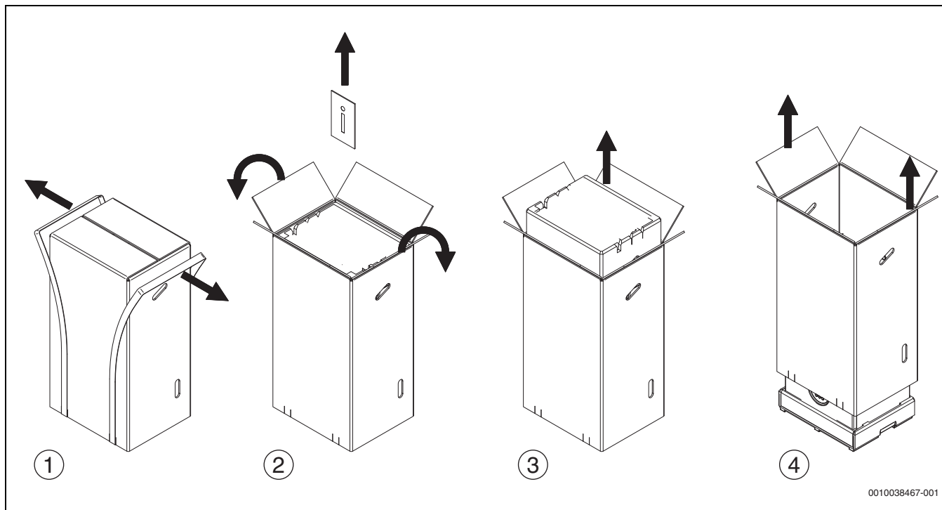
Rys. 32 Instrukcja rozpakowywania
