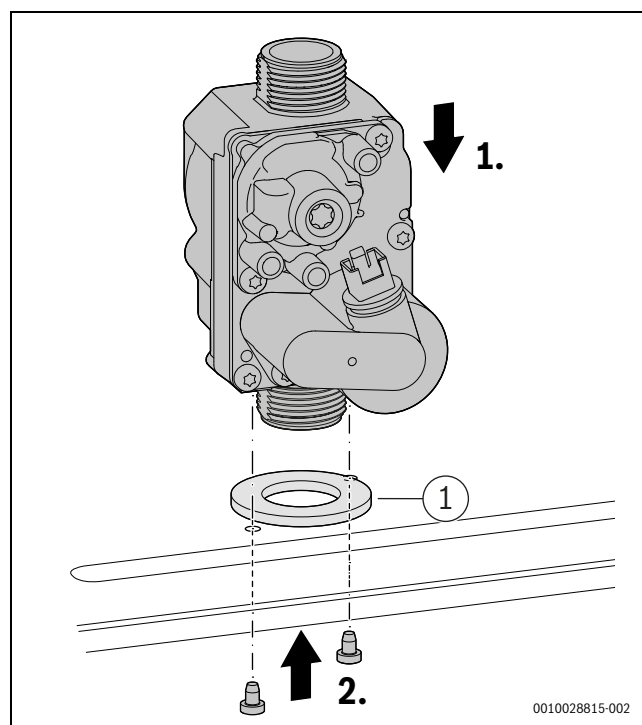
Rys. 76 Montaż armatury gazowej
