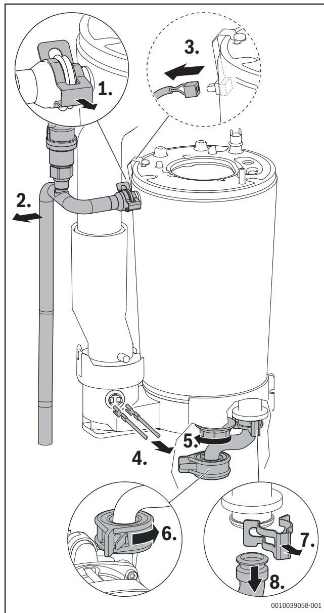
Rys. 66 Odłączanie rury zasilania, kabla i rury powrotu
