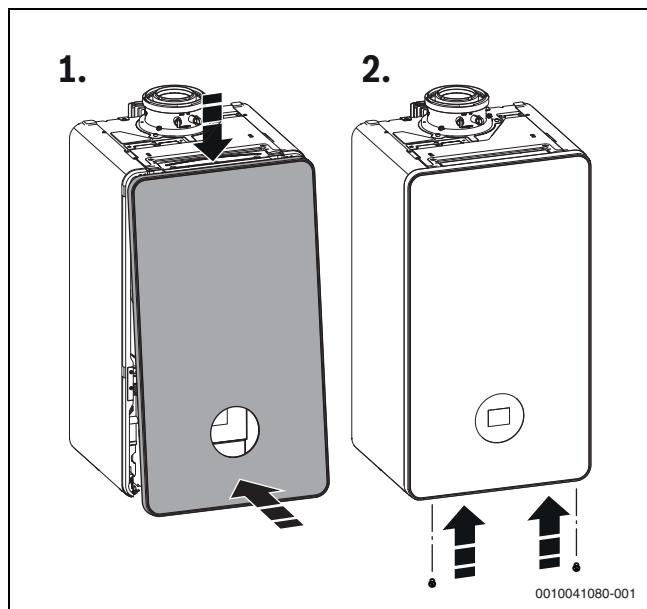
Rys. 43 Montaż obudowy
