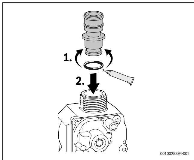
Rys. 78 Wkładanie dławika gazowego
