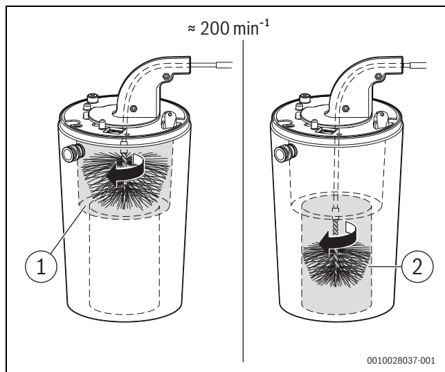
Rys. 62 Czyszczenie bloku ciepłego ( \approx 200 \text{ min}^{-1} , tylko ruch w prawo)
