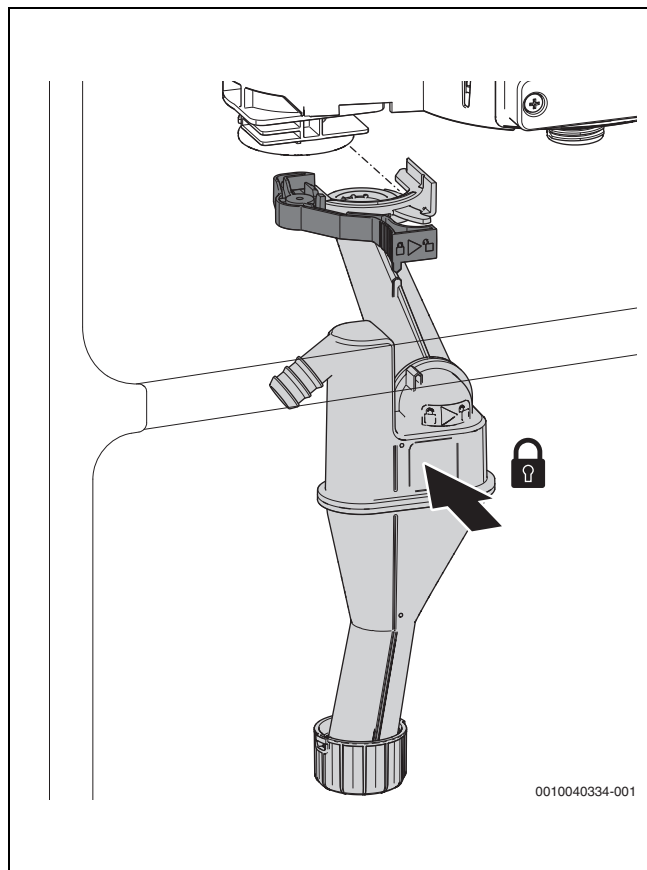
Rys. 85 Zakładanie syfonu kondensatu
