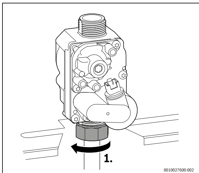
Rys. 74 Luzowanie nakrętki
