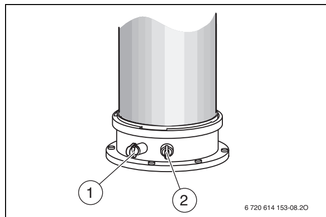
Rys. 48 Króćce pomiarowe spalin oraz powietrza do spalania
