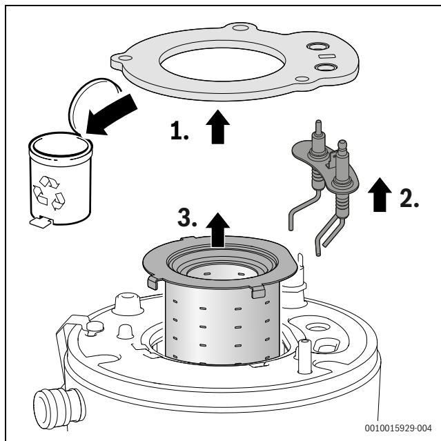
Rys. 57 Wyjmowanie palnika
