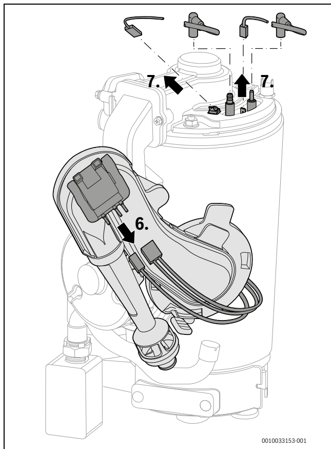
Rys. 53 Odłączanie kabli
