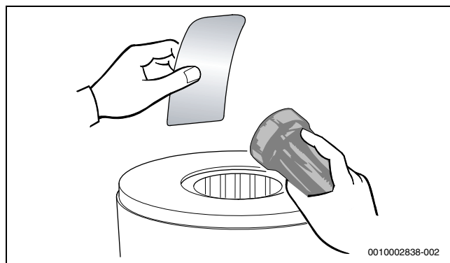
Rys. 64 Kontrola bloku ciepłego pod kątem pozostałości
