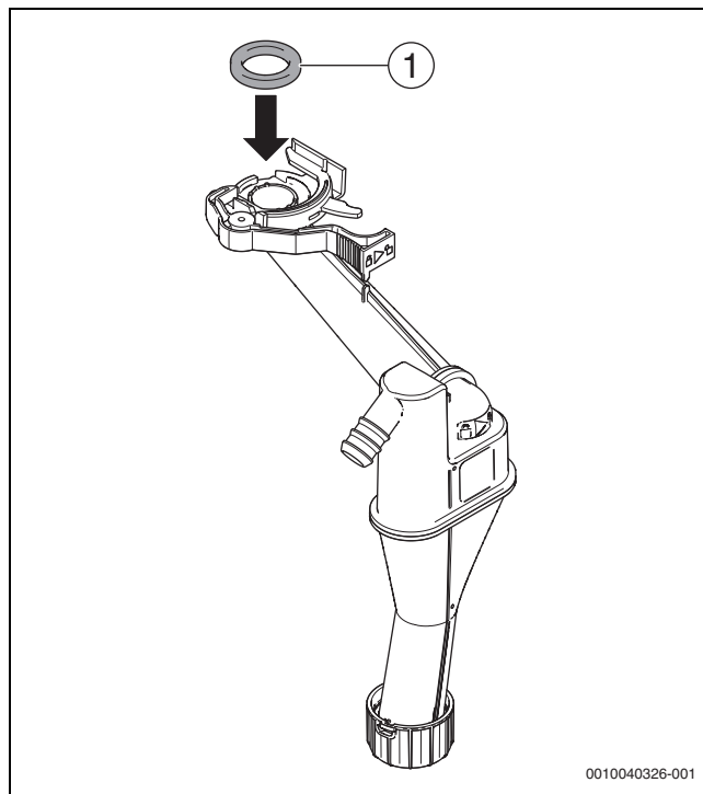
Rys. 83 Ułożenie nowej uszczelki na syfonie kondensatu
