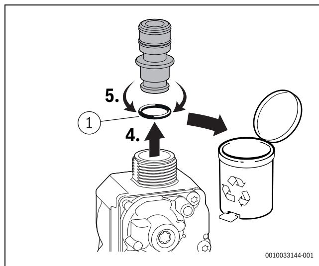
Rys. 73 Usuwanie dławika gazowego
