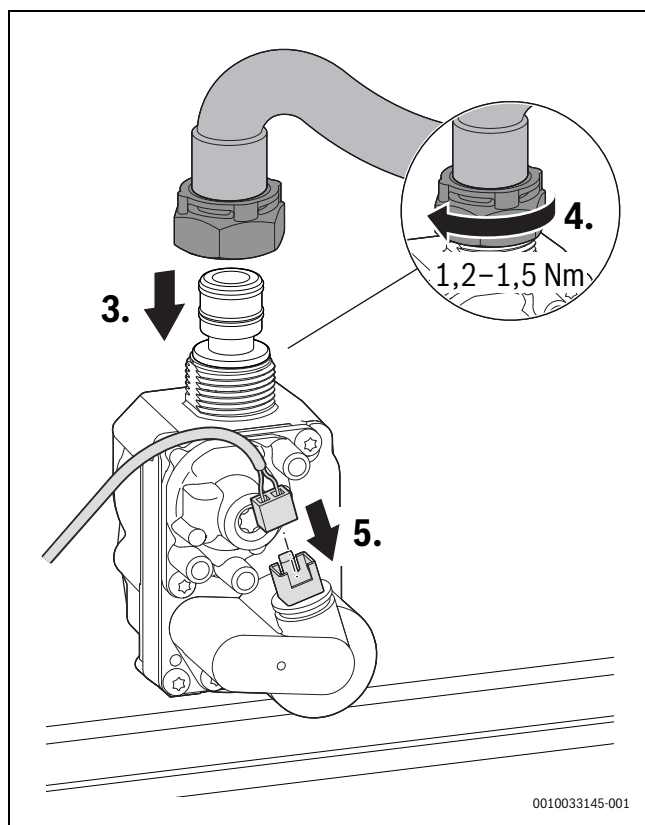
Rys. 79 Podłączanie węża gazowego i wtyczki – Przestrzeganie momentu dokręcenia
