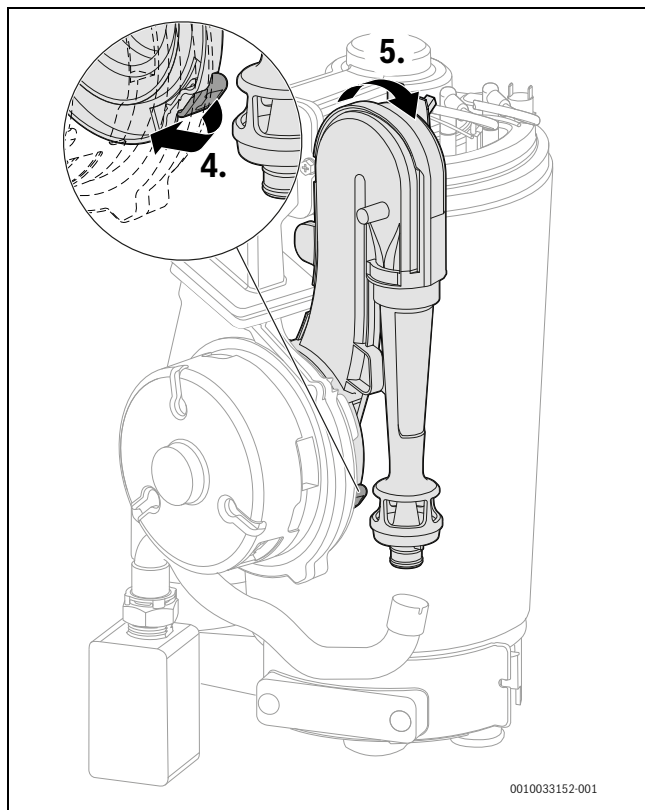
Rys. 52 Demontaż rurki Venturiego
