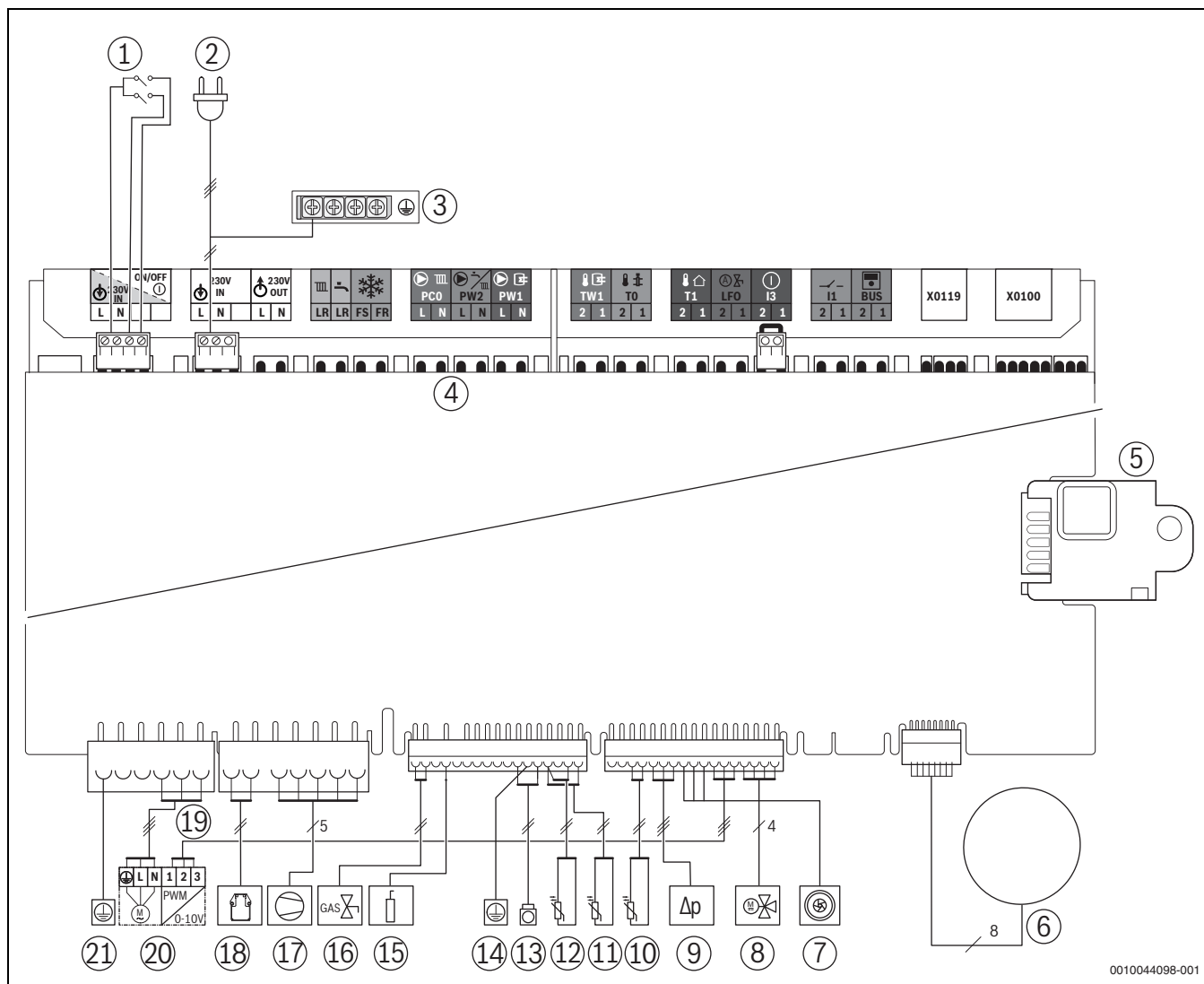
Rys. 91 Okablowanie elektryczne
