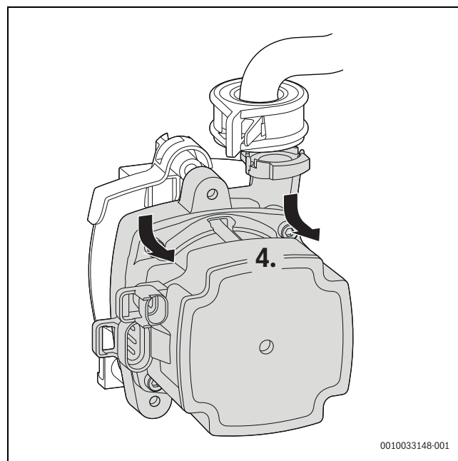
Rys. 70 Wyjmowanie pompy c.o.
