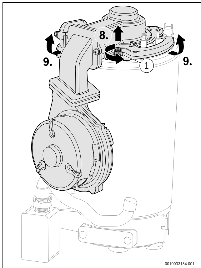
Rys. 54 Zdejmowanie pokrywy palnika z wentylatorem i z zespołem mieszającym
