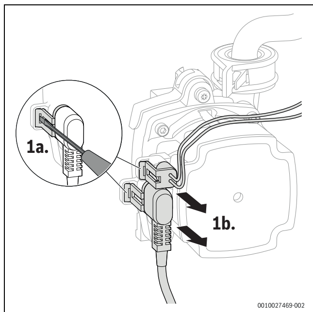
Rys. 68 Odłączanie wtyczki od pompy c.o.
