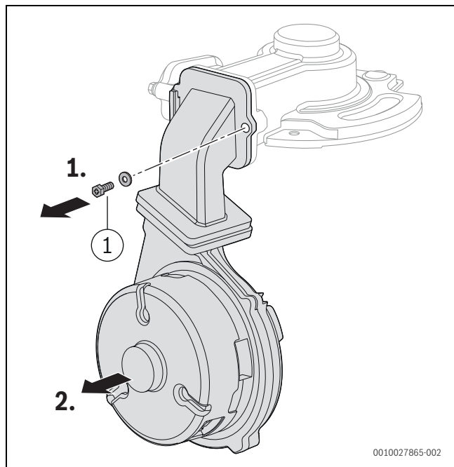
Rys. 55 Demontaż wentylatora i zespołu mieszającego
