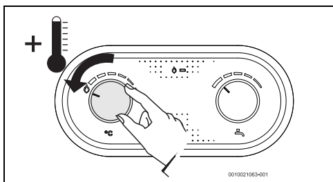
Rys. 7 Zwiększanie mocy
