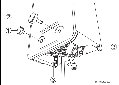
Rys. 16 Zdjąć obudowę
